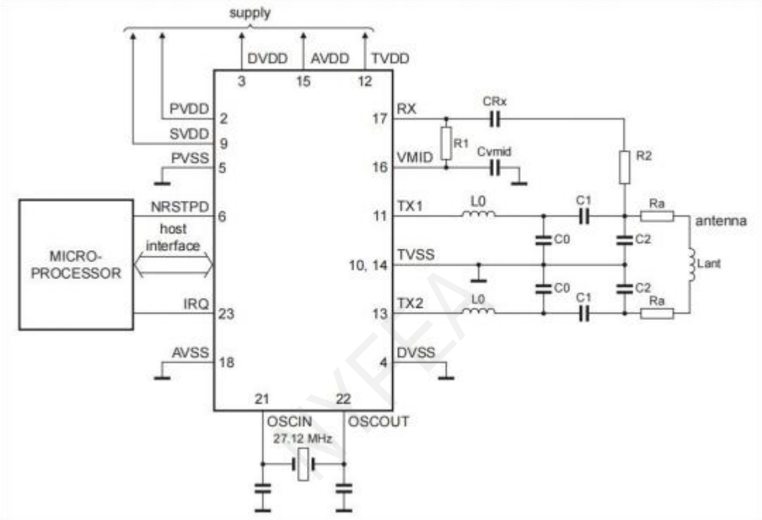
图 6-1 典型应用图
